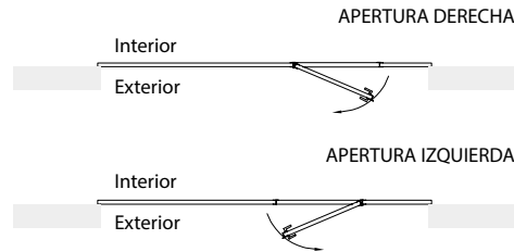
Puerta peatonal izquierda
