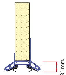
Para puertas de máximo hasta 4 m. de ancho de luz.
