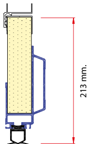
Para puertas de hasta 5 m. de ancho de luz.
