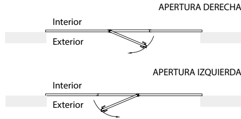
Puerta peatonal centrada
