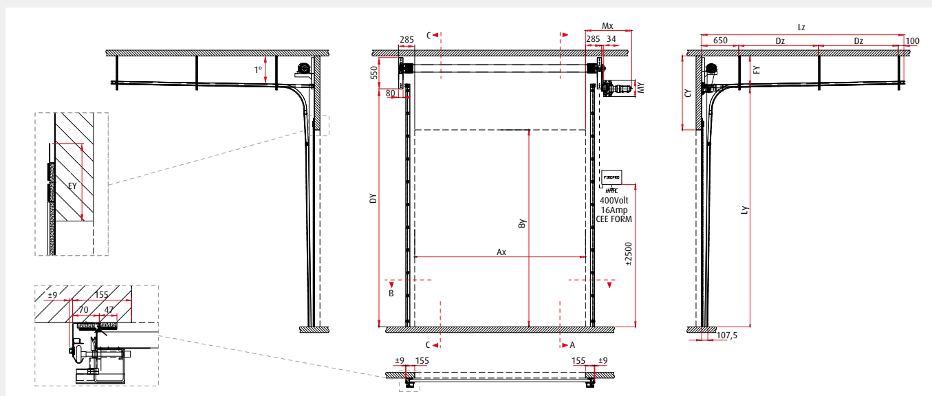
Medidas modelo EI-Secc' Cortafuegos 120'
